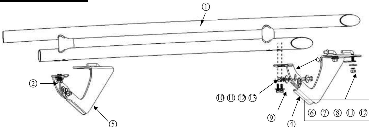
Left bracket-B
